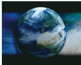
data_earth
